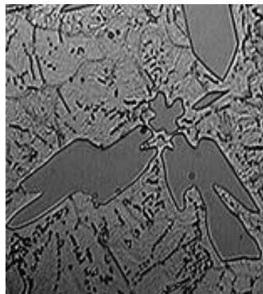
Microestrutura de liga metálica - 400x de aumento
